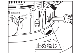
〈止めねじの場合〉
