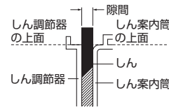
〈体止めねじの場合〉
