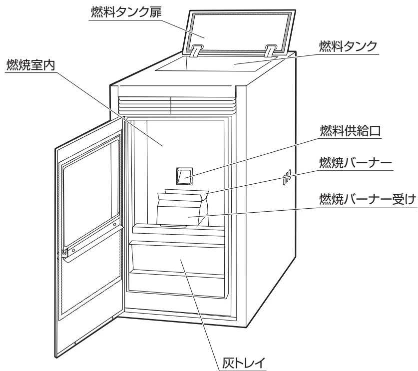
[内部構造図]
