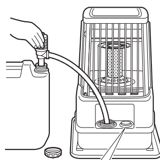
油量計
